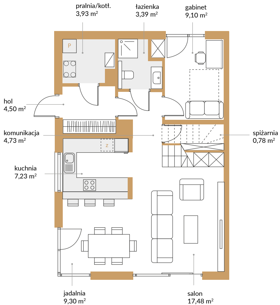
Parter: 60,44 m 2
